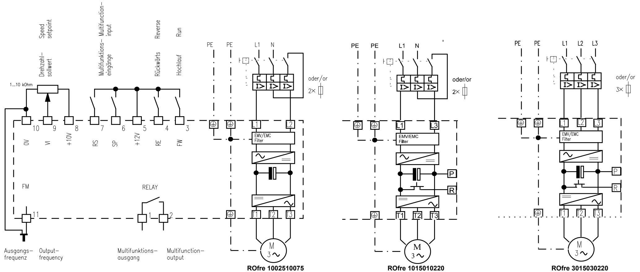
Bild 2.1: Grundanschlußplan ROfre 896
